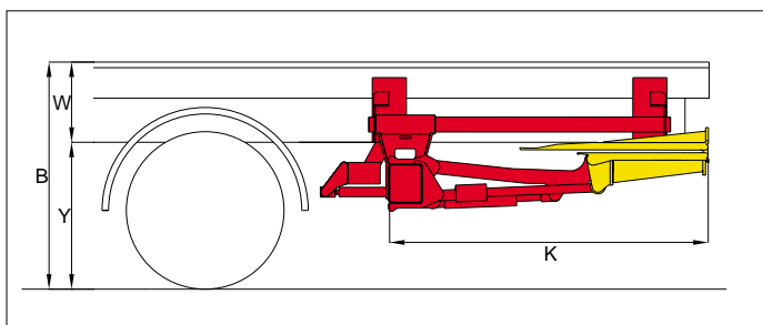
DVB 46 VE/1 - pedana a un piegamento
