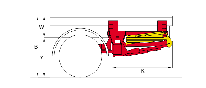
DVB 46 VE/2 - pedana a due piegamenti
